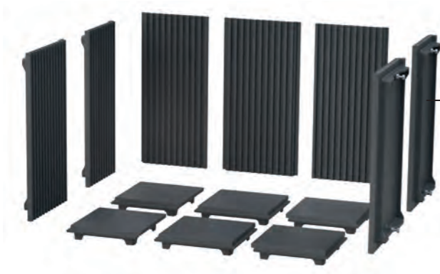
Foyer modulaire revêtu en fonte. Les panneaux de sol et les panneaux de protection coupe-feu ont une dimension de trame de 220 mm.
